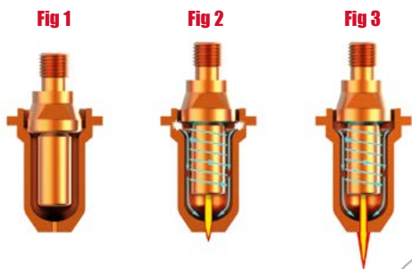
Fig 1: 在不工作时电极和割嘴的相对位置。
